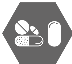
Interactions médicamenteuses
